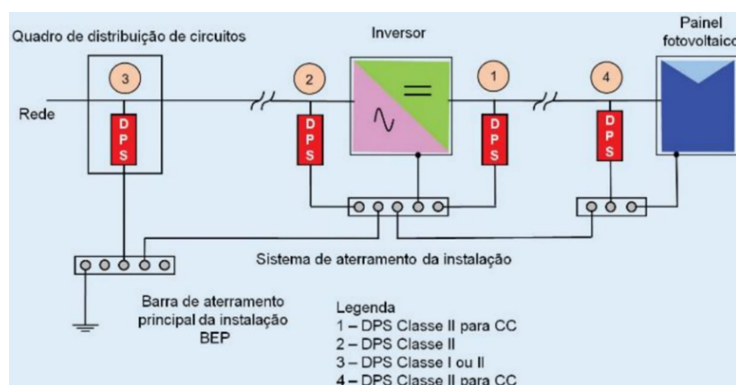
Figura 6: Localização dos DPS (Fonte: PAULINO, 2016)
